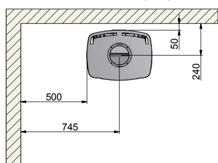
65-2, 65-4, 65-8 og 65-10 (med sideglas) Parallel installation på bagvæg
