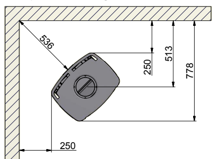
65-2, 65-4, 65-8 og 65-10 (med sideglas) 45° hjørneopstilling:
