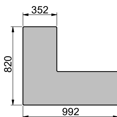
Lille formgulvplade i klart eller røgfarget glas
