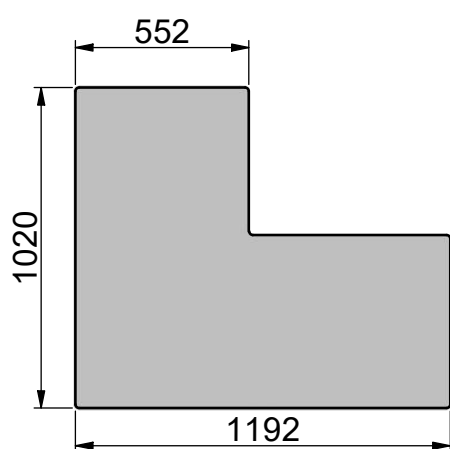
Stor formgulvplade i klart eller røgfarget glas
